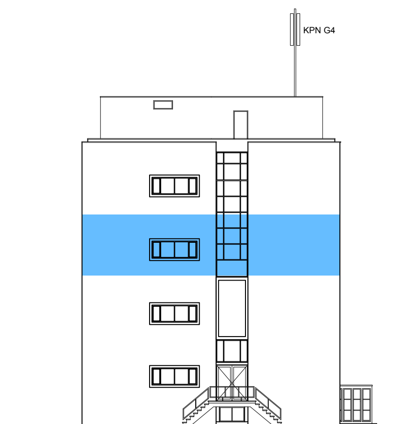
Rechter zijgevel
