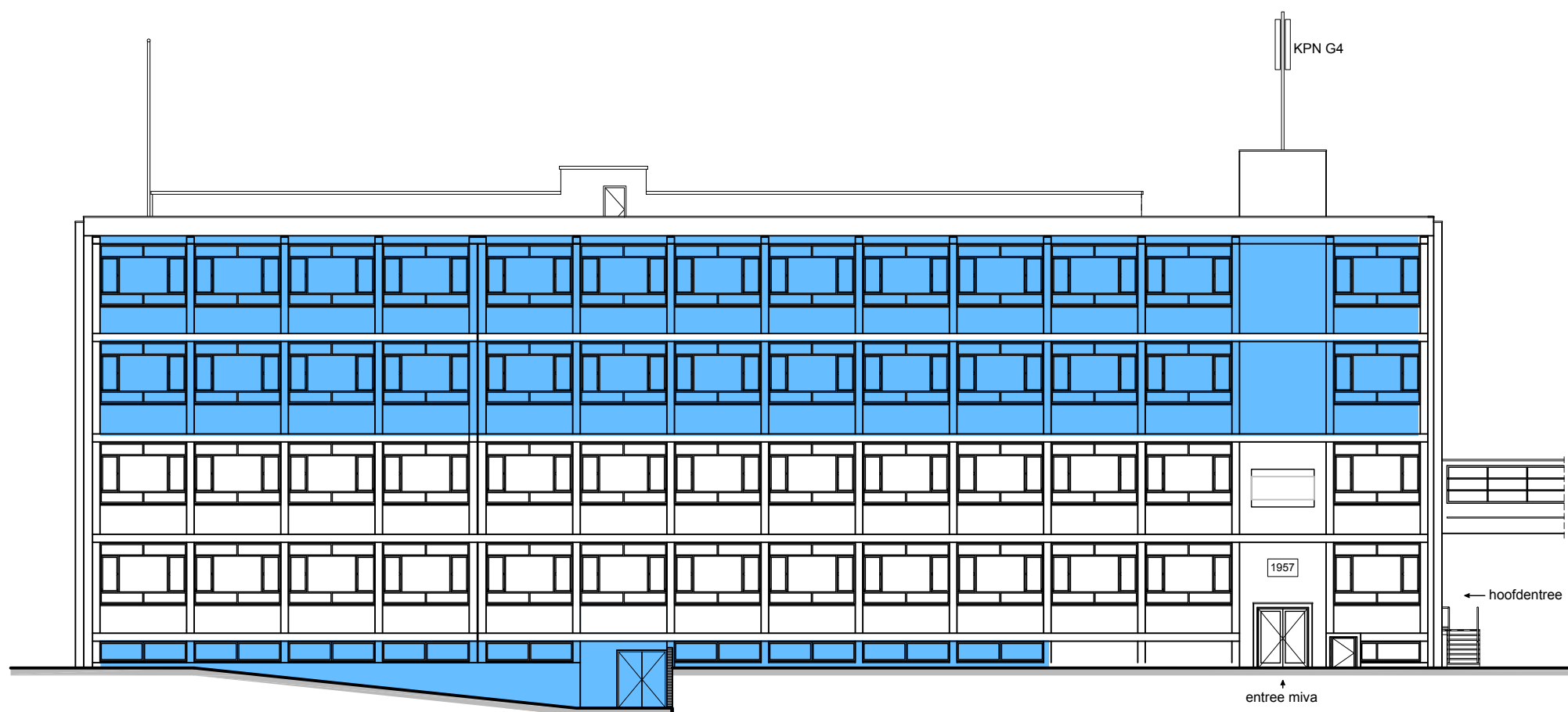
Voorgevel
