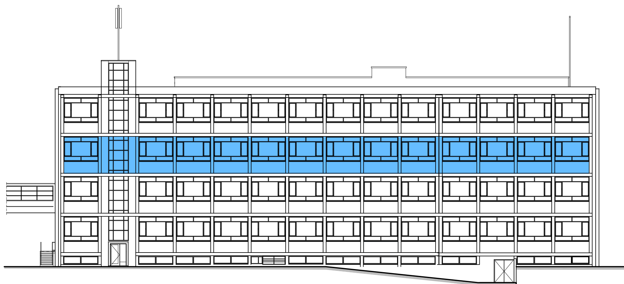
Achtergevel
