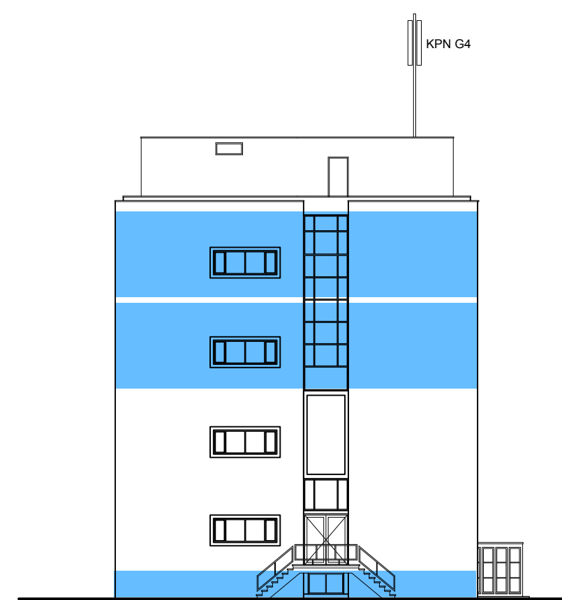
Rechter zijgevel
